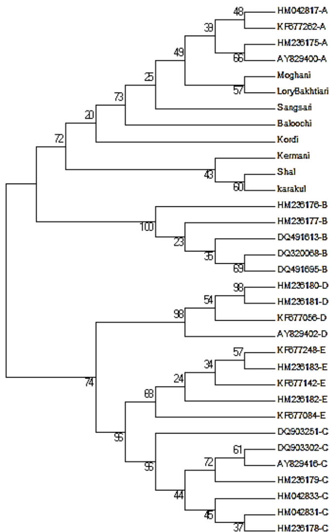
شکل ۳- قسمتی از مقایسه نتایج توالی‌یابی ناحیه HVR-III میتوکندری گوسفندان بومی ایران Figure 3- Partial sequence comparison of HVR-III region from Iran's native sheep
