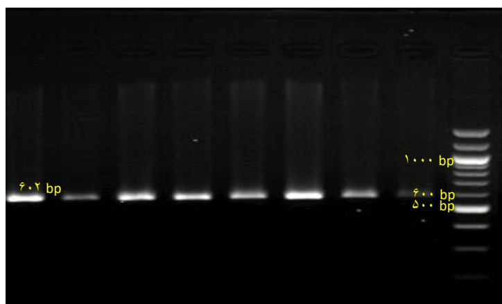
شکل ۱ - الکتروفورز محصولات واکنش زنجیره‌ای پلیمراز ژن‌های D-Loop Figure 1- Electrophoresis of the PCR products of the D-Loop gene
